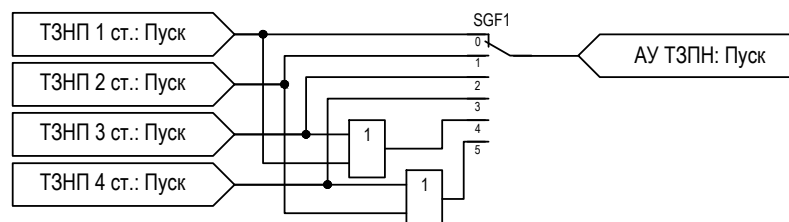
Рисунок 2.32 – Функциональная схема АУ ТЗНП
